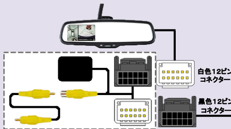
純正オプションバックカメラ
