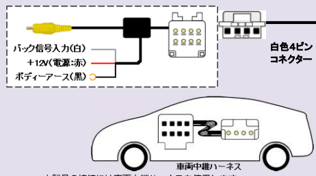
ディーラーオプション バックカメラ
