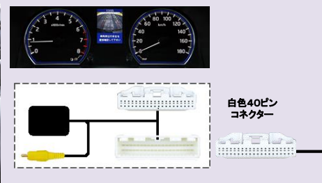
純正オプションバックカメラ
