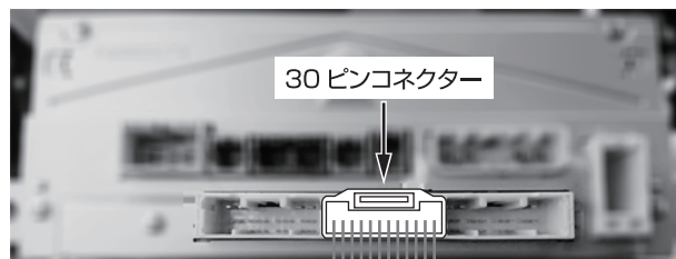
ディスプレイオーディオ（オーディオユニット）裏側
