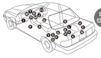
取付位置図
