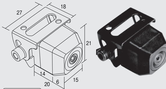
寸法図(単位mm)
